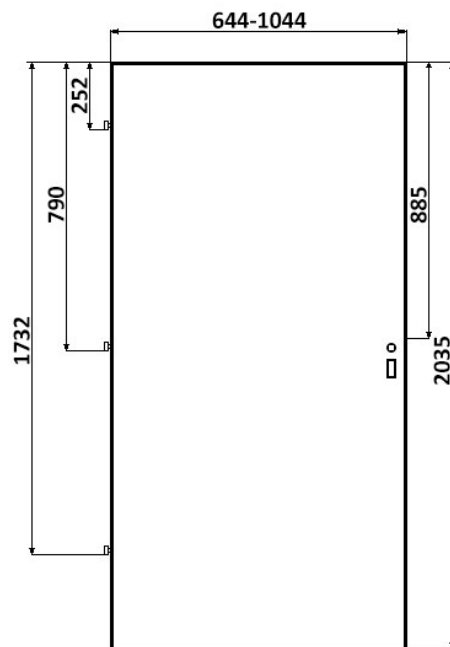
Rysunek 1. Wymiary zewn. skrzydła
